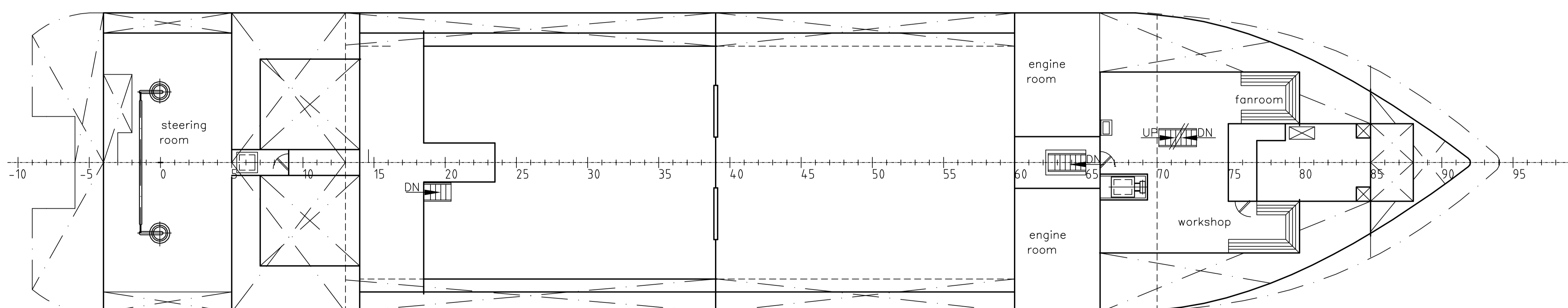
TWEENDECK
