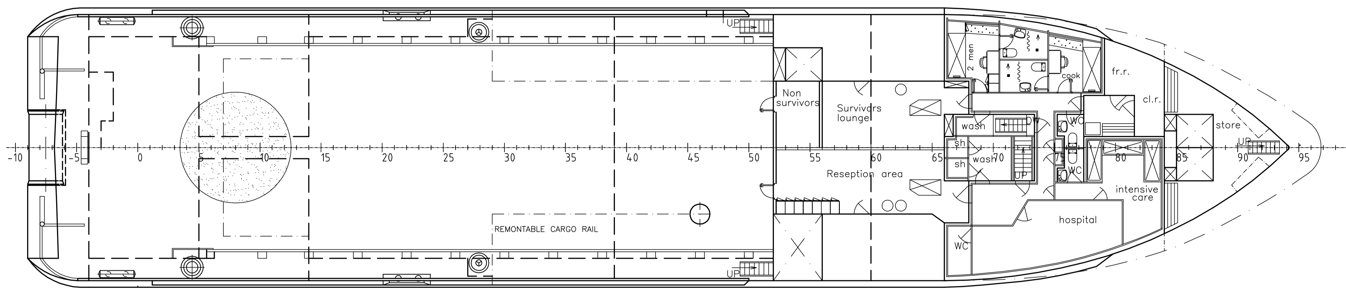
MAINDECK
